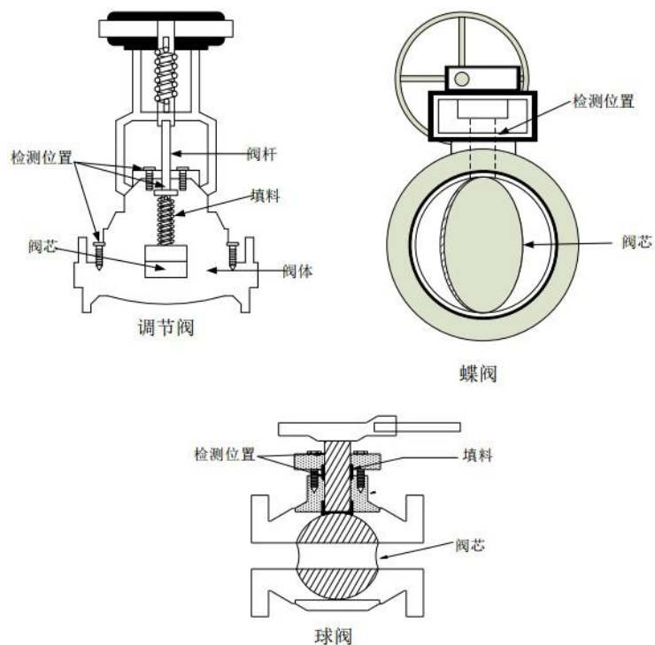
图 5.5-4 调节阀、球阀和蝶阀检测位置
