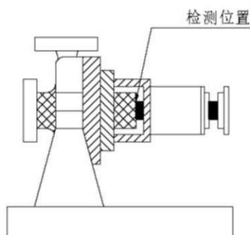
图 5.5-5 离心泵轴检测位置
