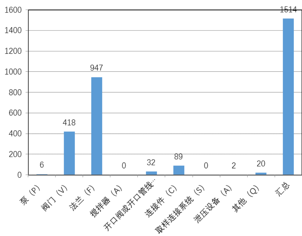
图 3.3.7 火炬系统总检测密封点情况
