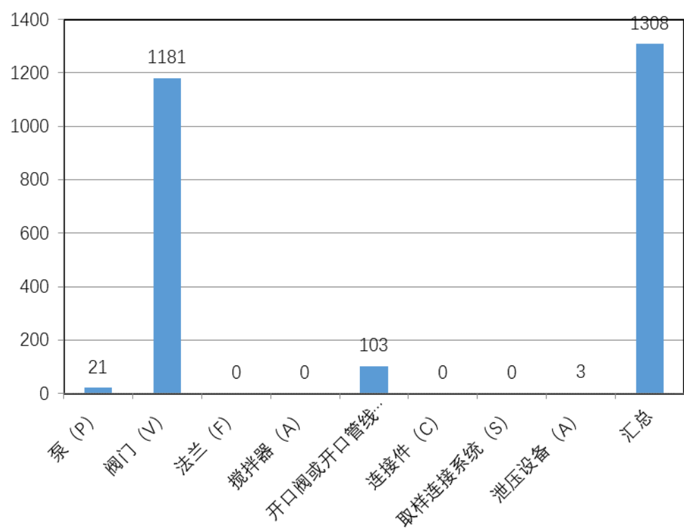
图 3.3.4 4万吨/年环氧丙烷装置总检测密封点情况
