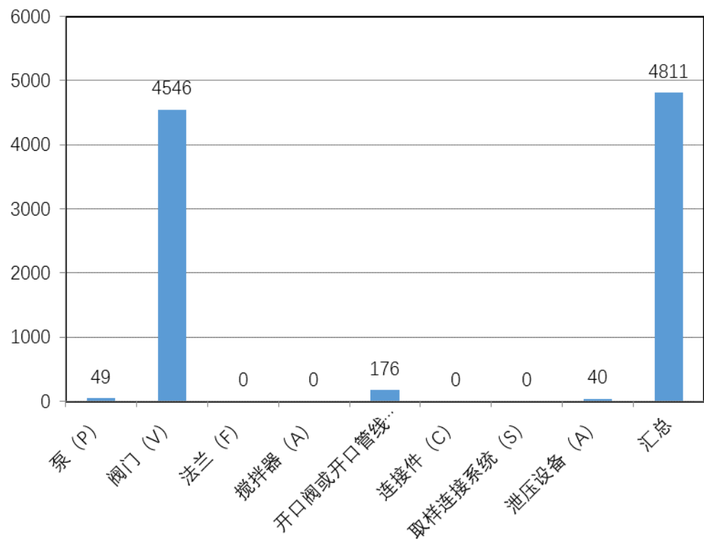
图 3.3.5 20 万吨/年混合碳四深加工装置总检测密封点情况
