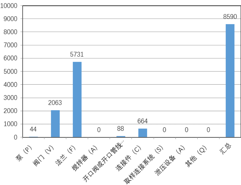
图 3.3.11 30 万吨/年电解液装置总检测密封点情况
