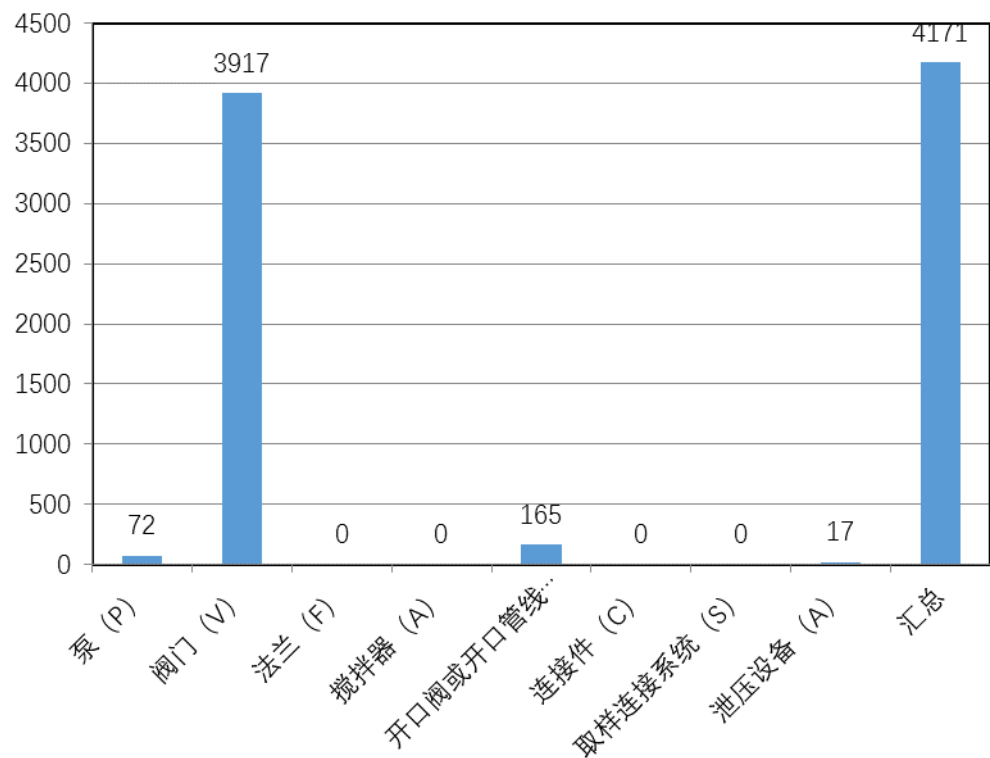
图 3.3.6 罐区（储运）总检测密封点情况
