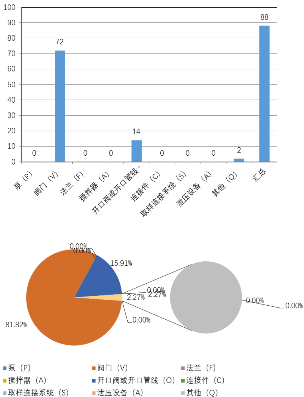
图 4.3.1 TVA2020 仪器(FID)复测范围点数分布图
