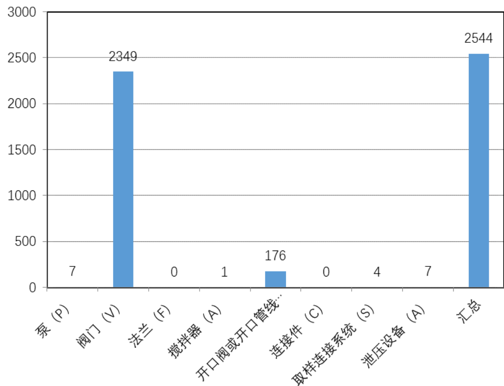
图 3.3.8 4.3 万吨/年乙碳装置总检测密封点情况
