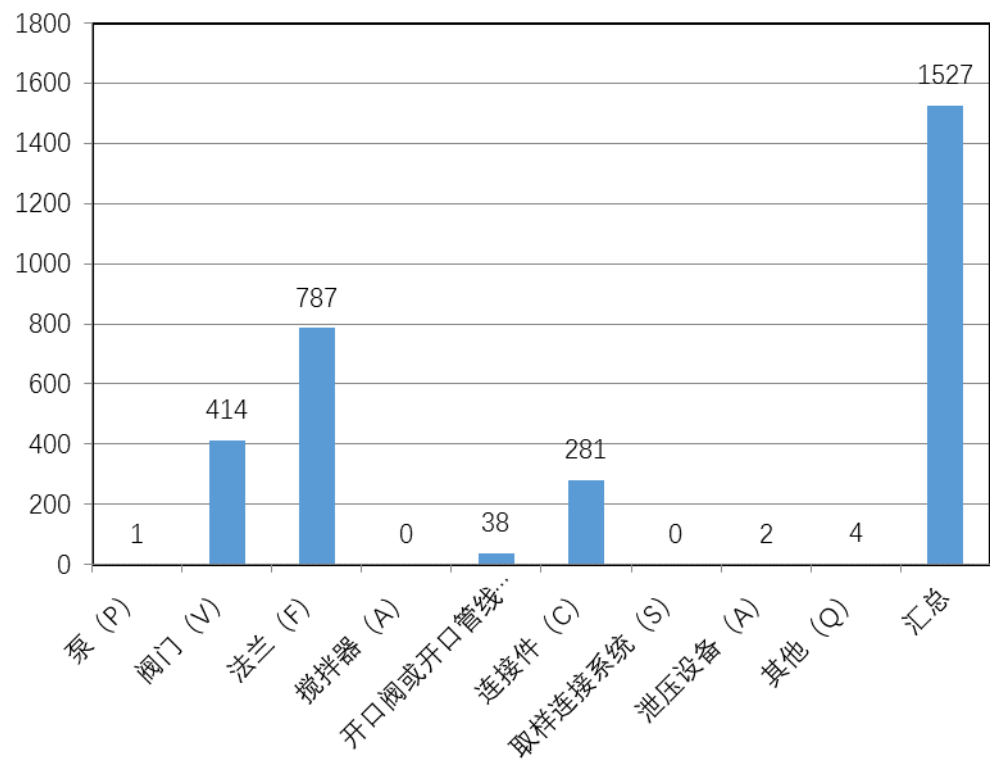
图 3.3.10 焚烧炉总检测密封点情况
