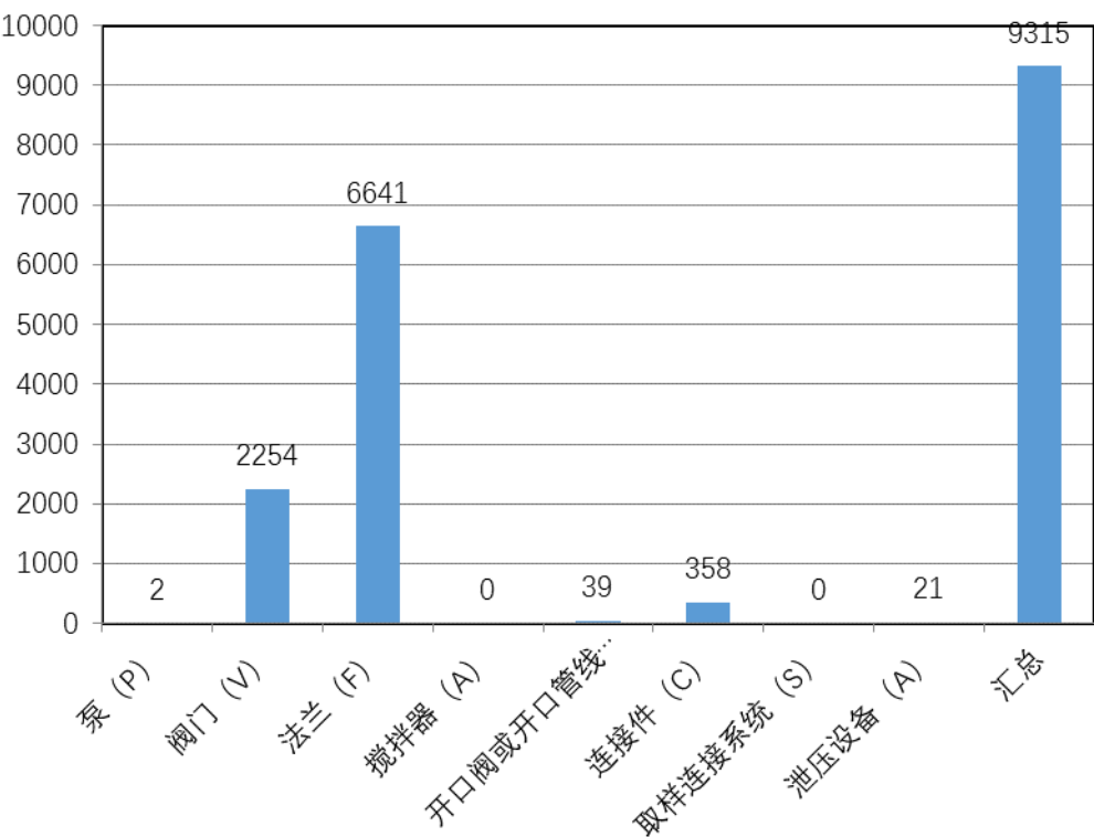
图 3.3.9 1.1 万吨/年添加剂装置总检测密封点情况
