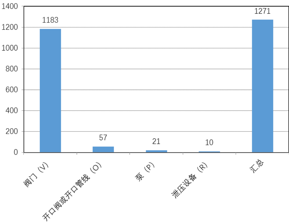
图 3.3.2 甲醇钠装置总检测密封点情况
